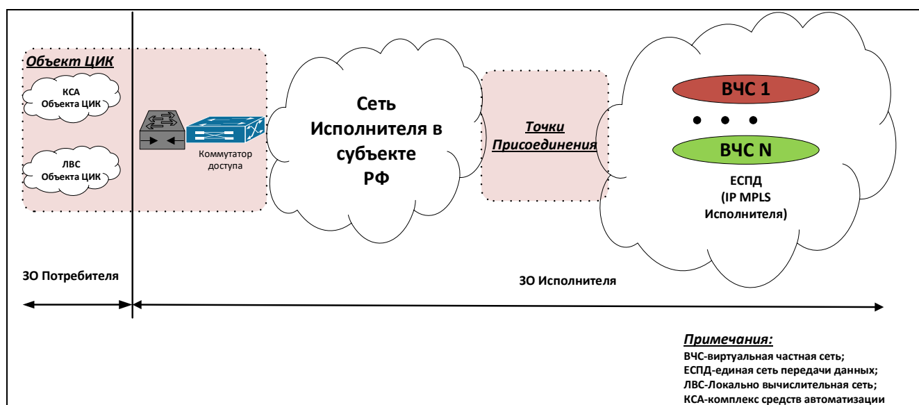
Рис.3. Архитектура Компонента Услуг связи «Передача данных».
